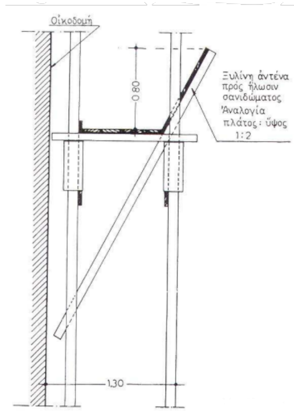
Εικ. 4 Εγκάρσια τομή του προστατευτικού προστεγάσματος
